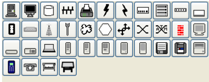
Abbildung 6.9: Netzwerk
