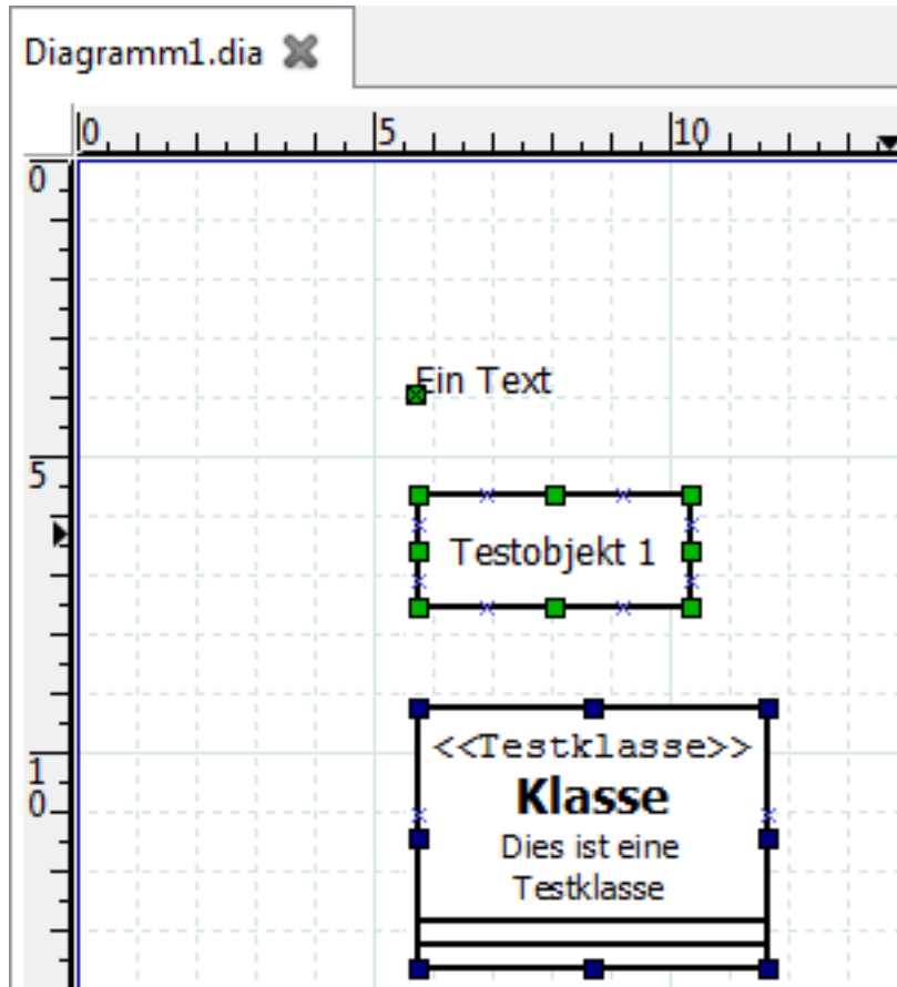
Abbildung 4.20: Linksbündig ausgerichtet
