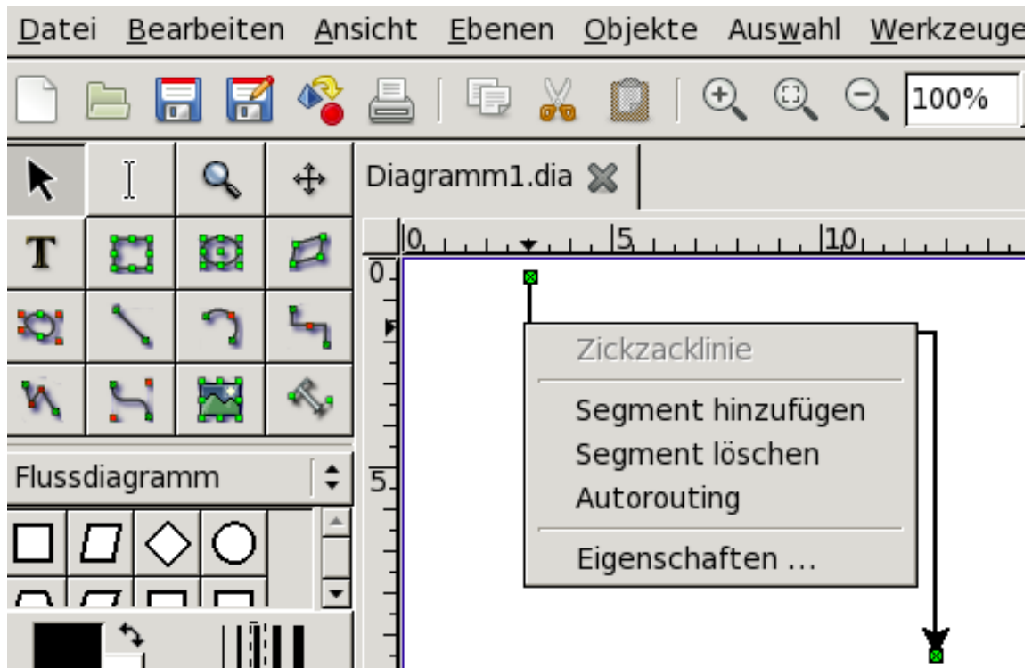
Abbildung 5.2: Kontextmenü Zickzacklinie
