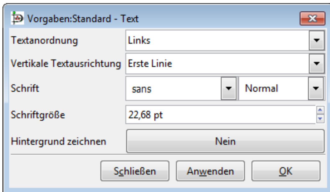
Abbildung 4.34: Vorgaben Texteeigenschaften
