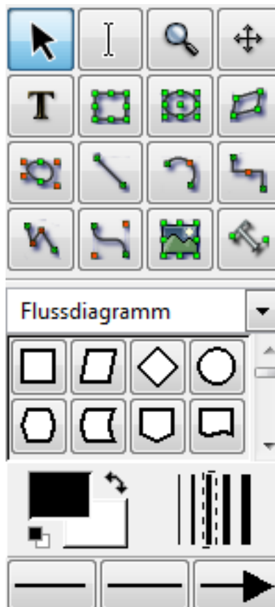
Abbildung 4.1: Dias Werkzeugkasten
