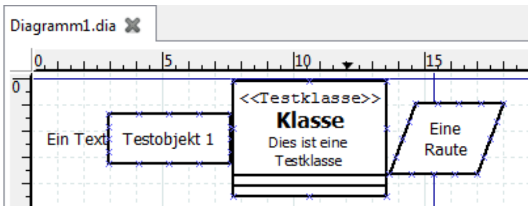
Abbildung 4.31: Ausrichtung / Angrenzend
