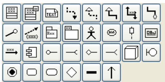
Abbildung 6.10: UML
