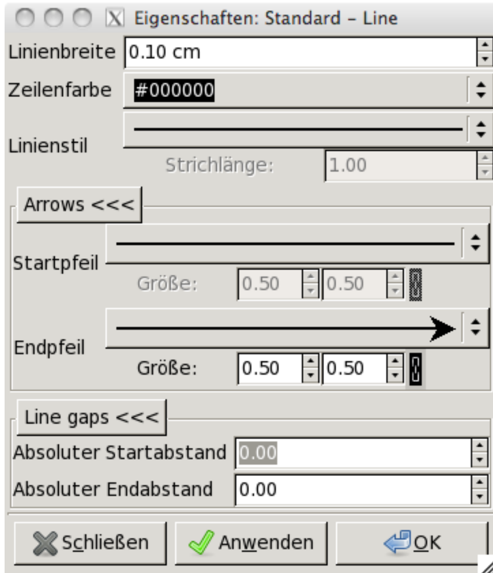
Abbildung 5.5: Linieneigenschaften
