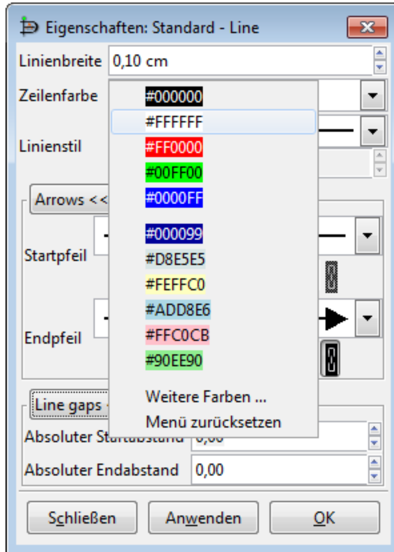
Abbildung 4.36: Farbauswahlliste
